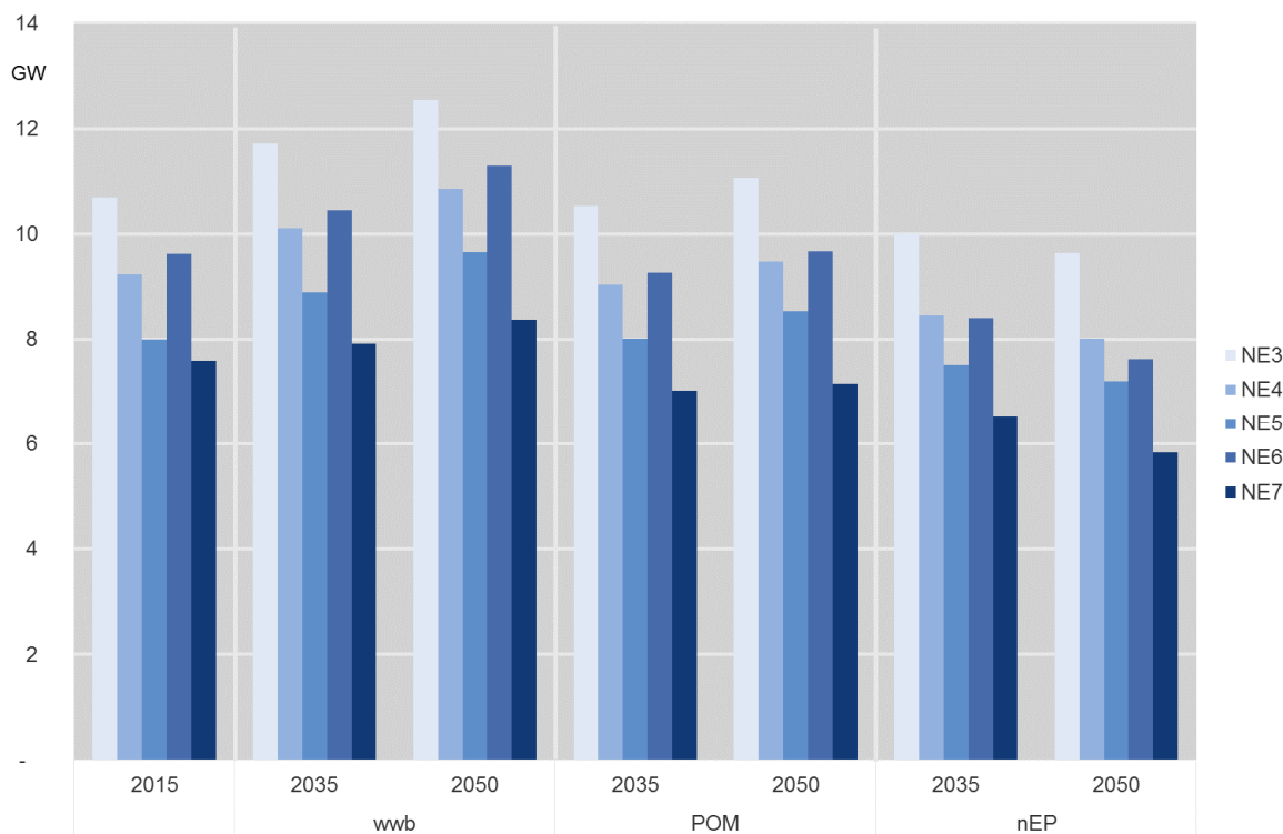
Bild 2.2: Jahreshöchstlasten (in GW) der jeweiligen Netzebenen in den drei Nachfrageszenarien wvb, POM und nEP in 2035 und 2050 im Vergleich zu 2015
